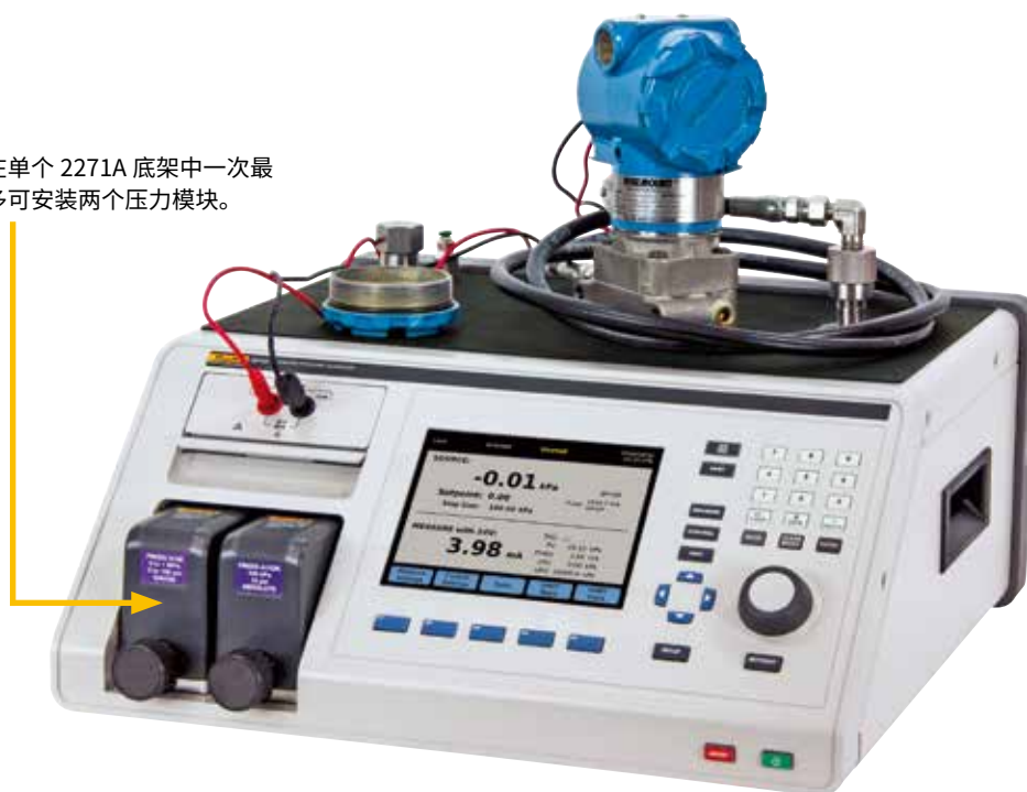
使用 2271A 对 4-20 mA 设备（例如该变送器）进行闭环、全自动校准。
