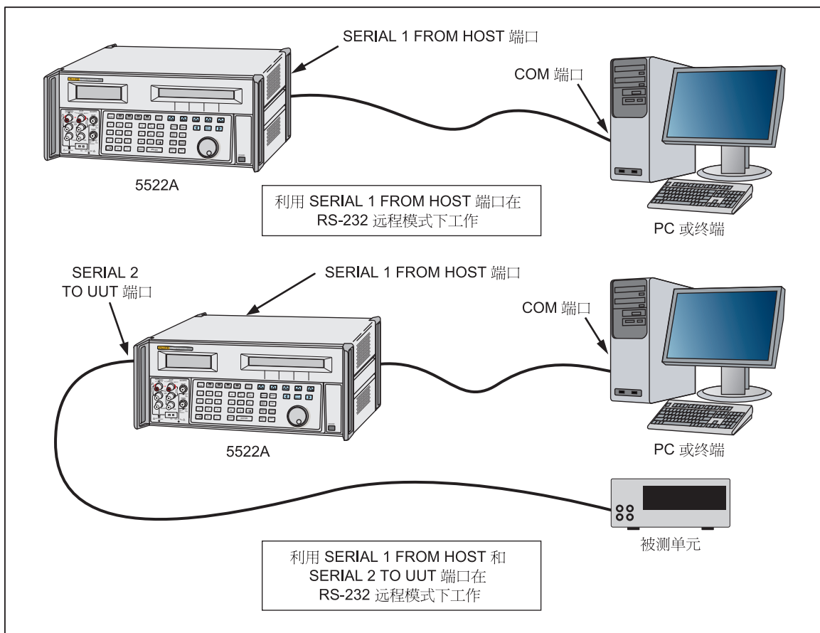
图 2.RS-232 远程连接
