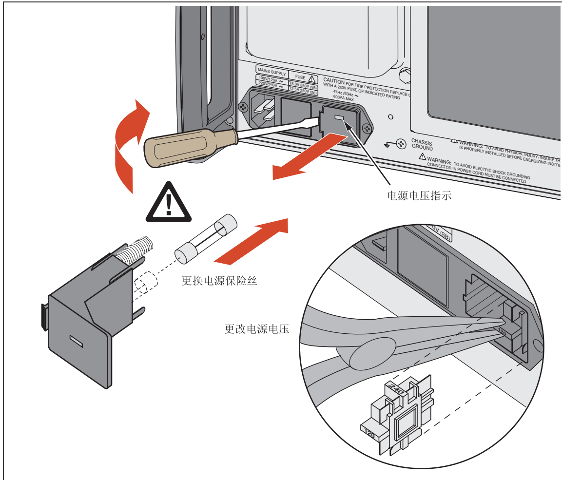
图 3. 如何拆卸保险丝及选择电源电压
