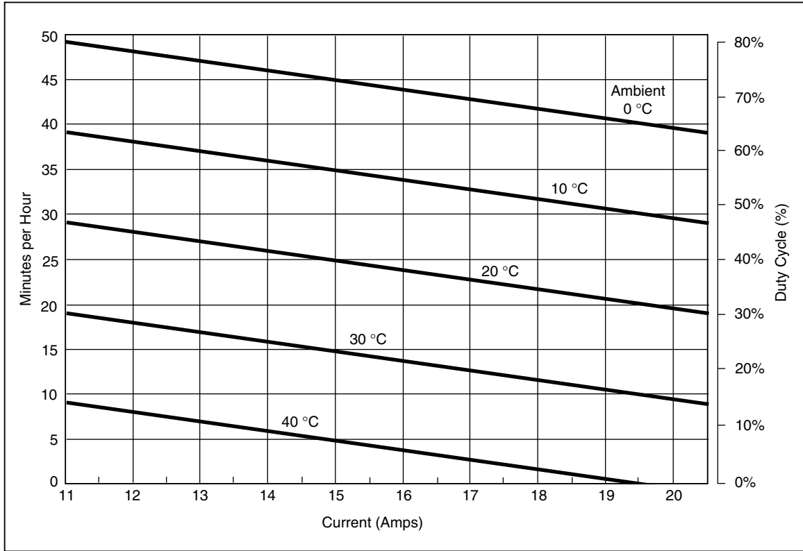
图 5. 电流 > 11 A 时的允许周期
