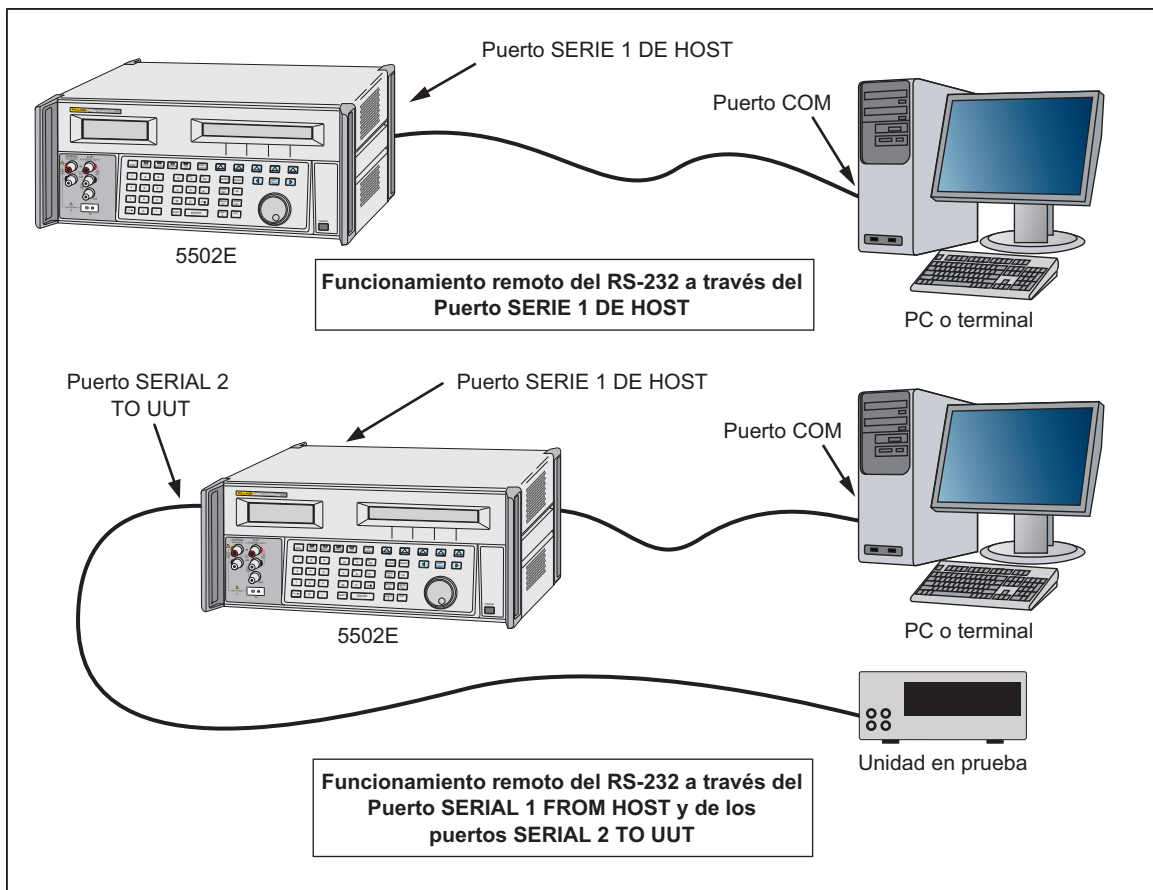
Figura 2. Conexión remota RS-232
