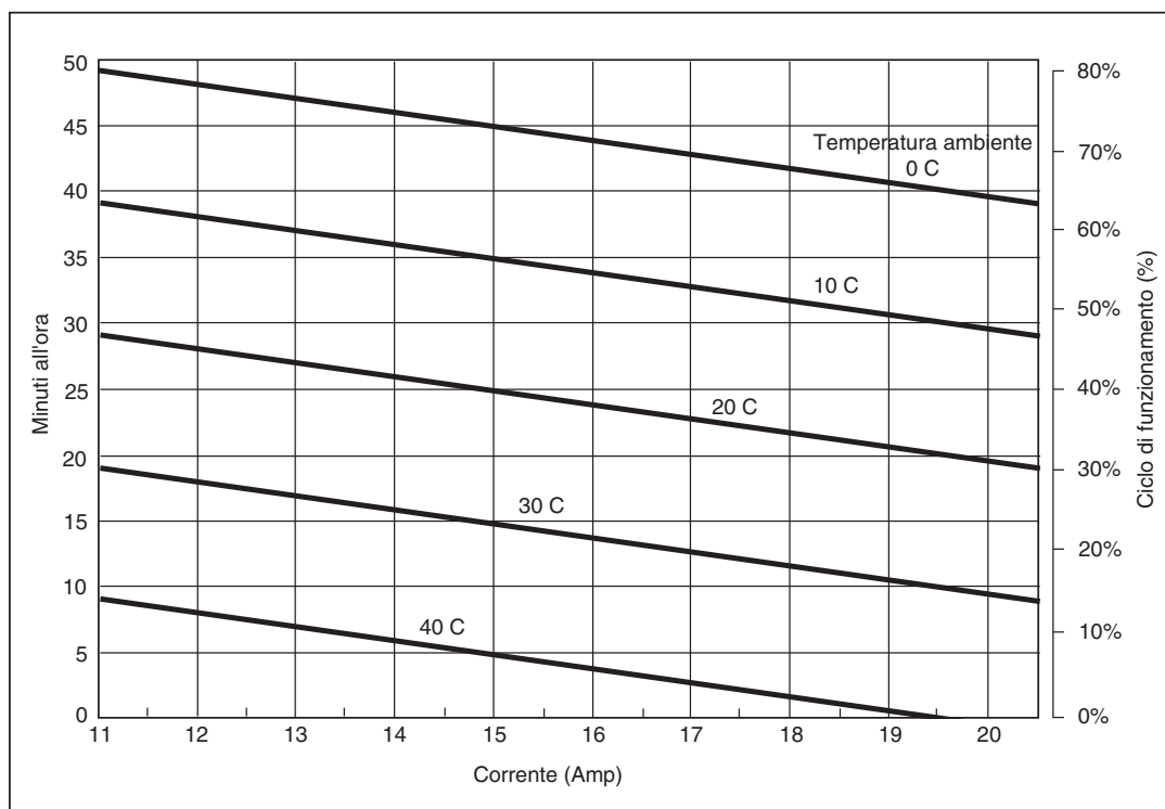
Figura 5. Durata di corrente consentita &gt; 11 A
