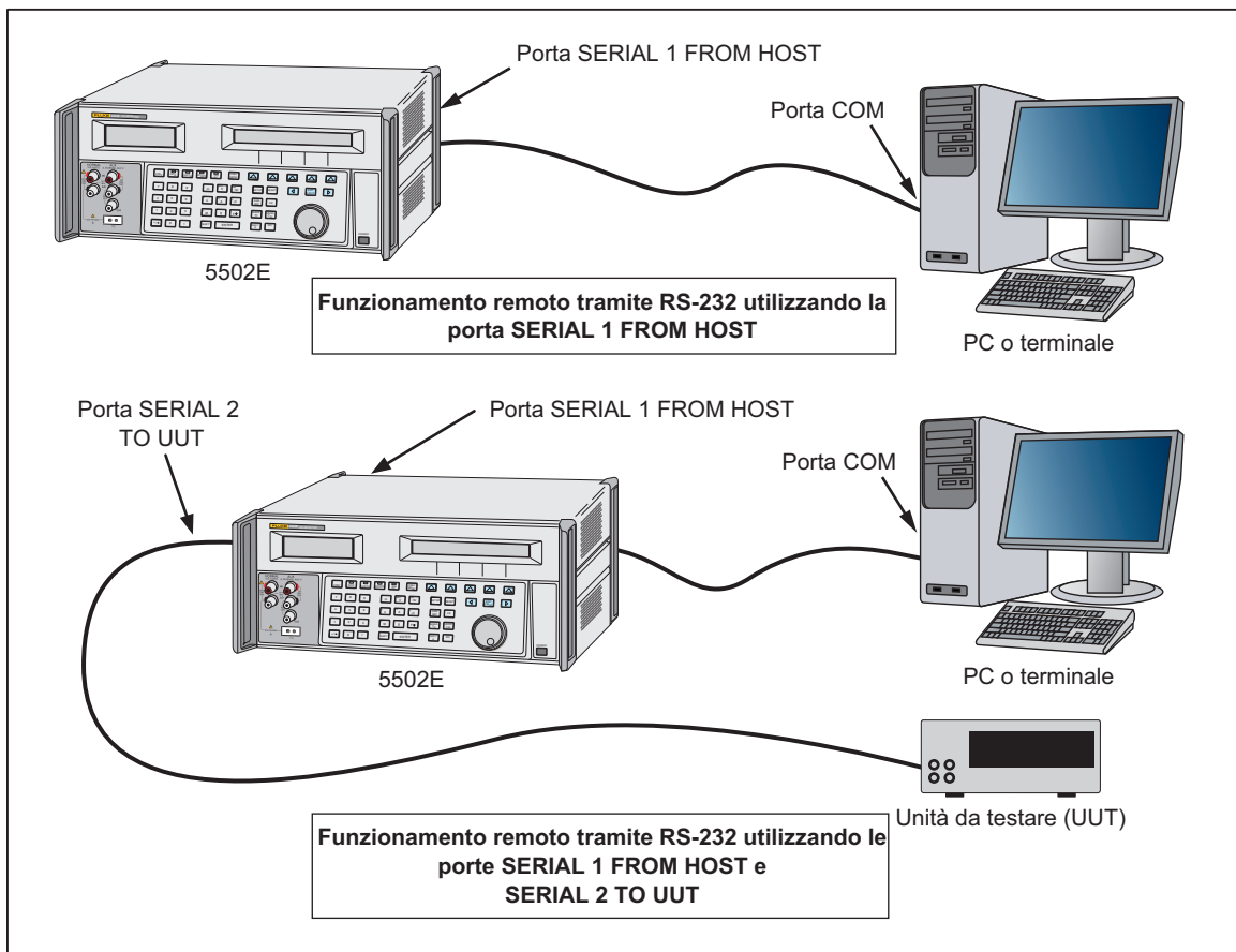
Figura 2. Funzionamento remoto tramite RS-232
